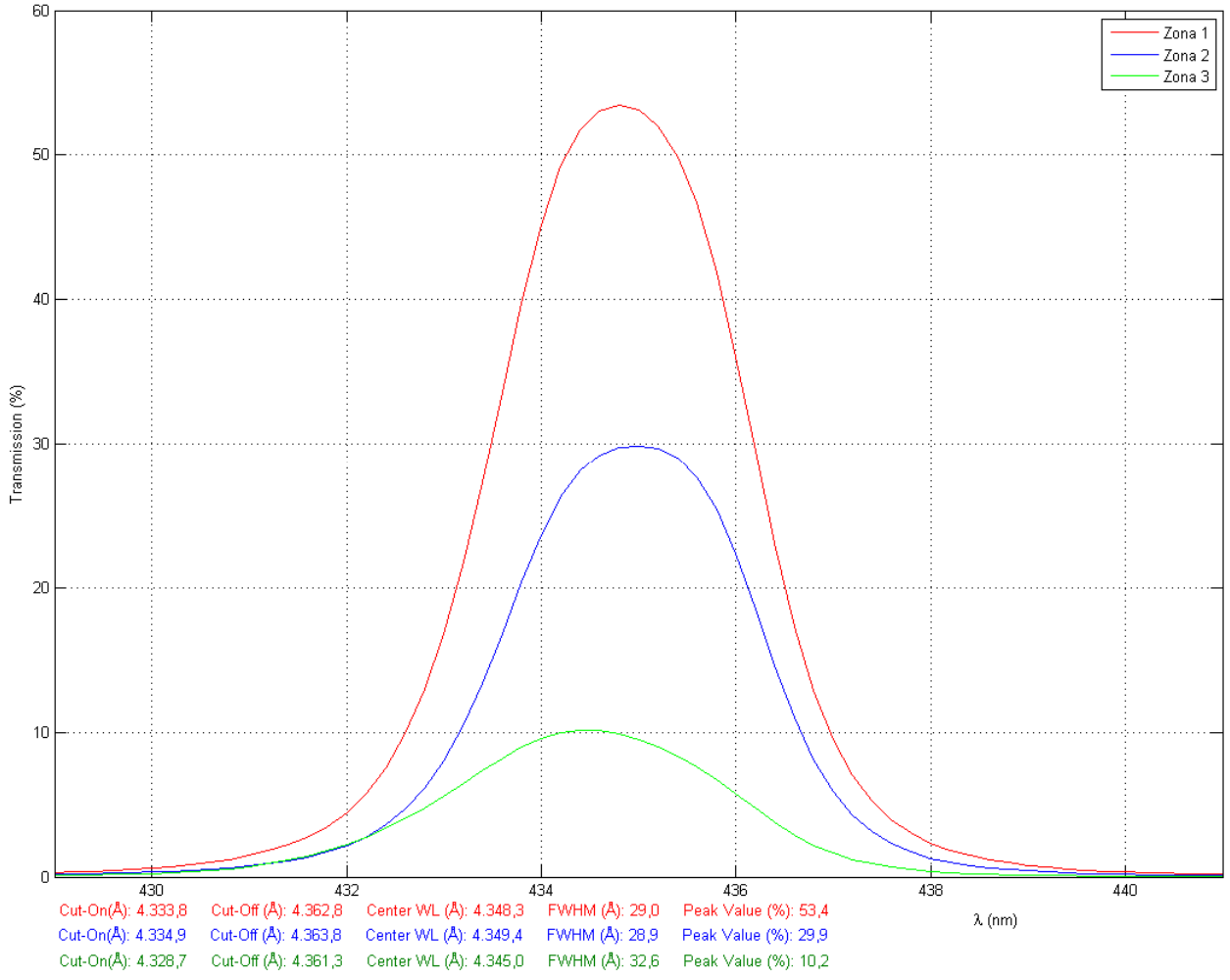
Líneas de Emisión H gamma, 4340/30
