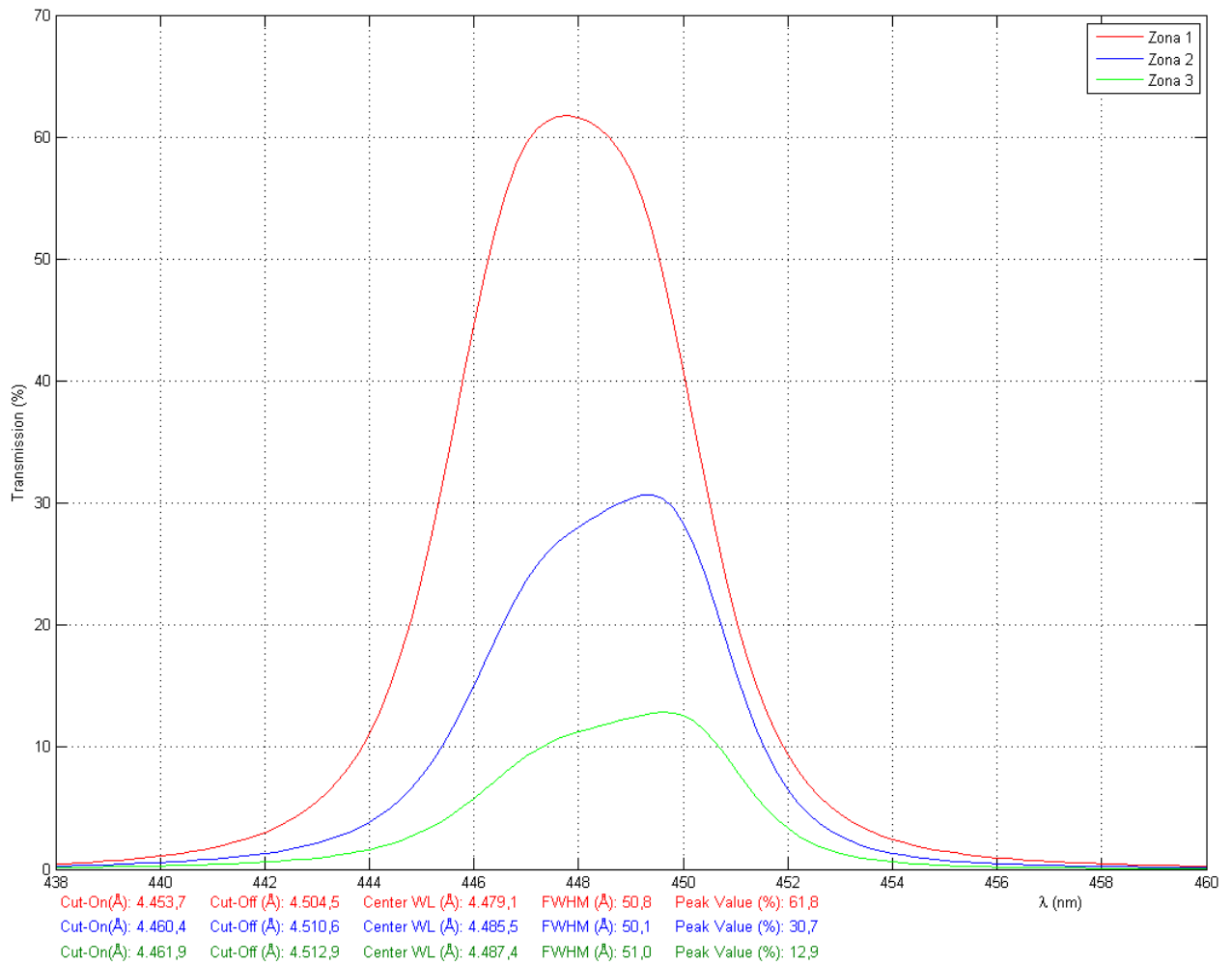
Líneas de Emisión Hel, 4471/50
