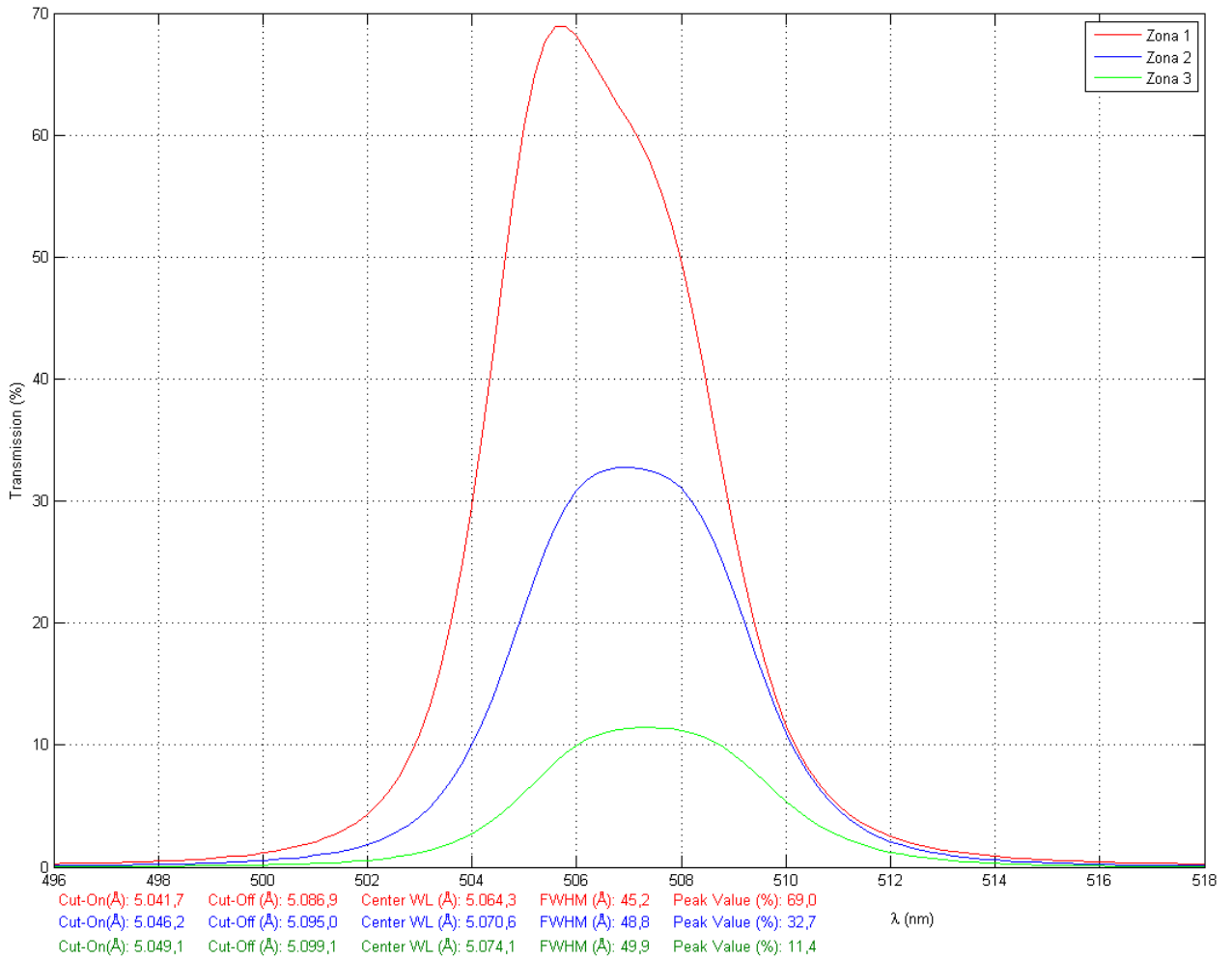
Líneas de Emisión OIII, 5057/50
