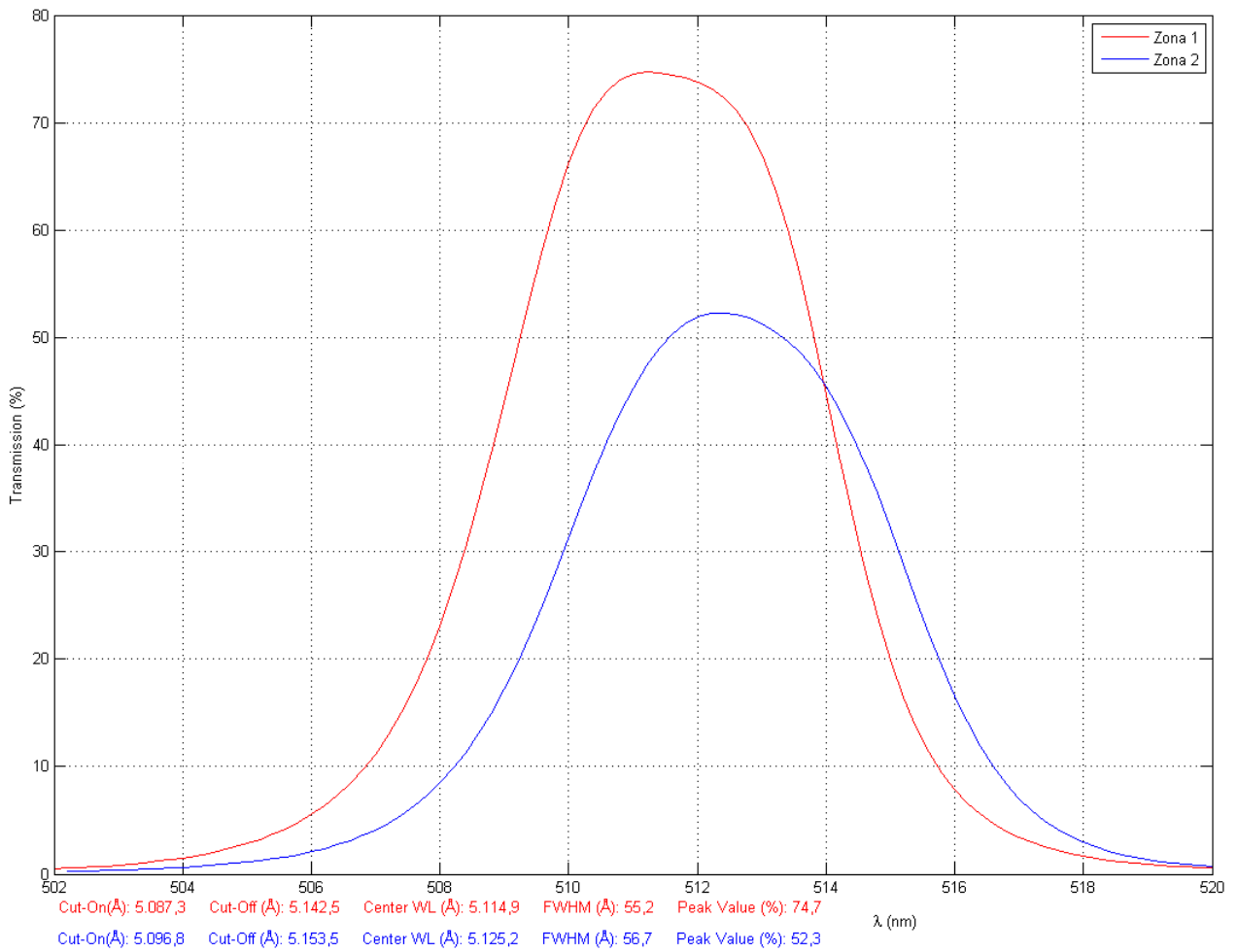
Líneas de Emisión OIII, 5107/50
