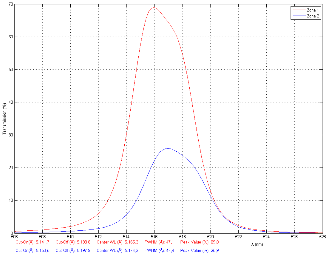
Líneas de Emisión OIII, 5157/50
