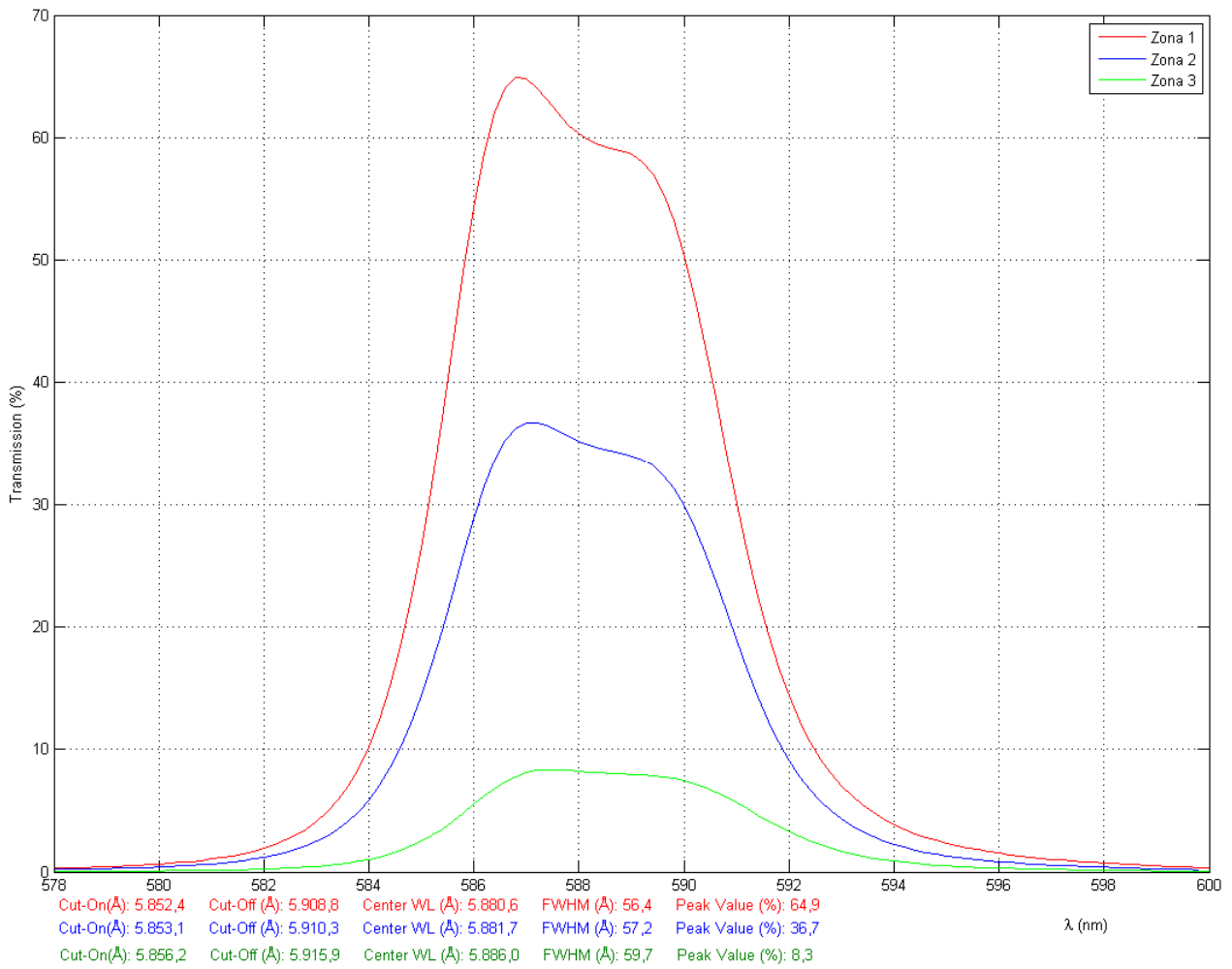
Líneas de Emisión Hel, 5876/50
