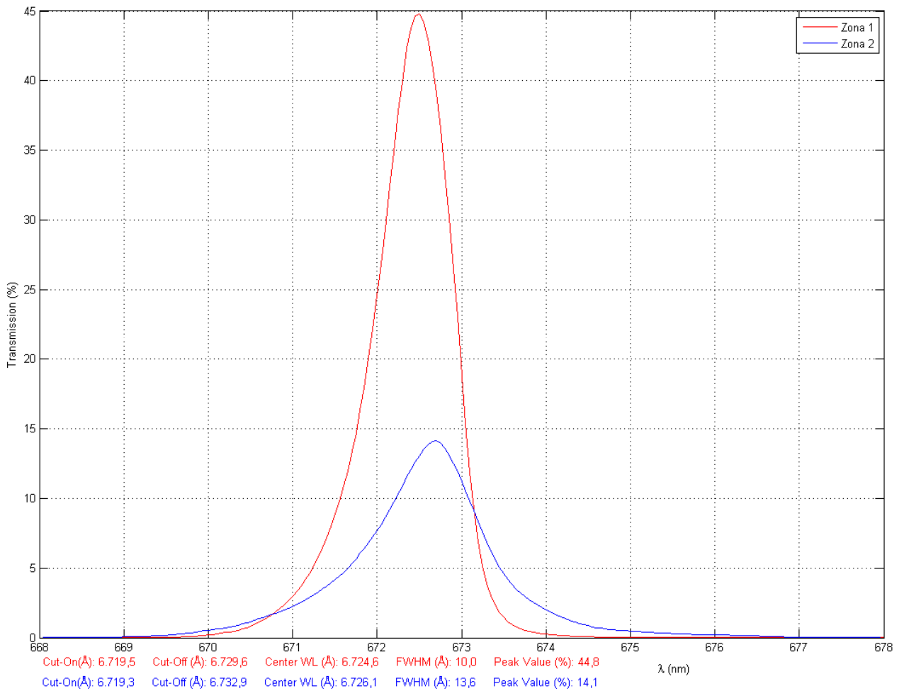
Líneas de Emisión SII, 6731/5
