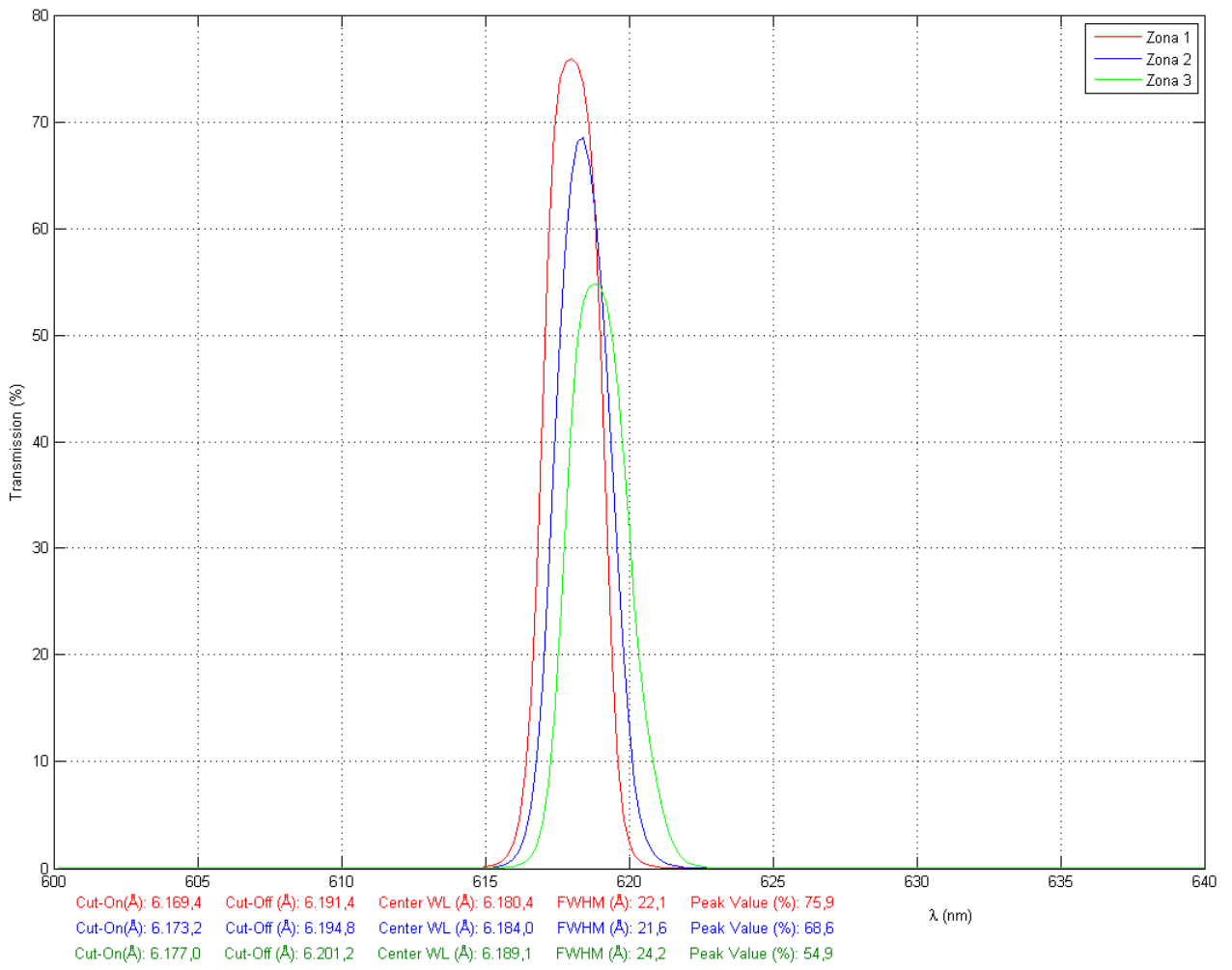
Bandas Moleculares, 6184/20
