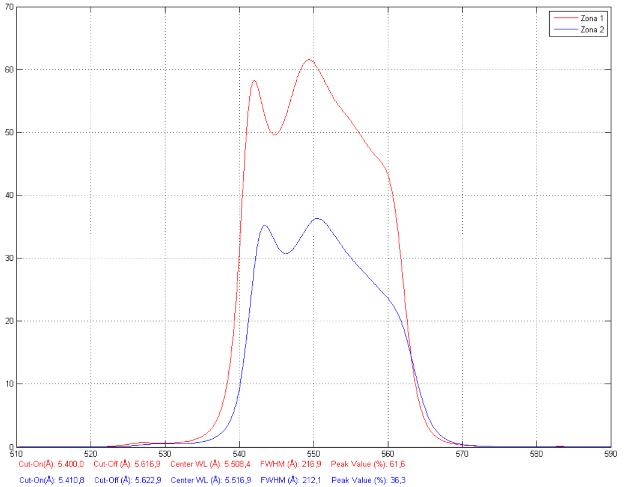
y Strömgren
